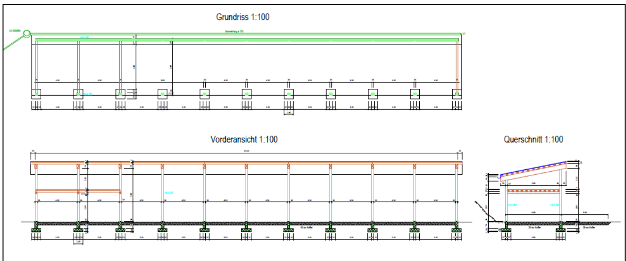
Vesta frontala, transversala e plan horizontal dalla remisa planisada
